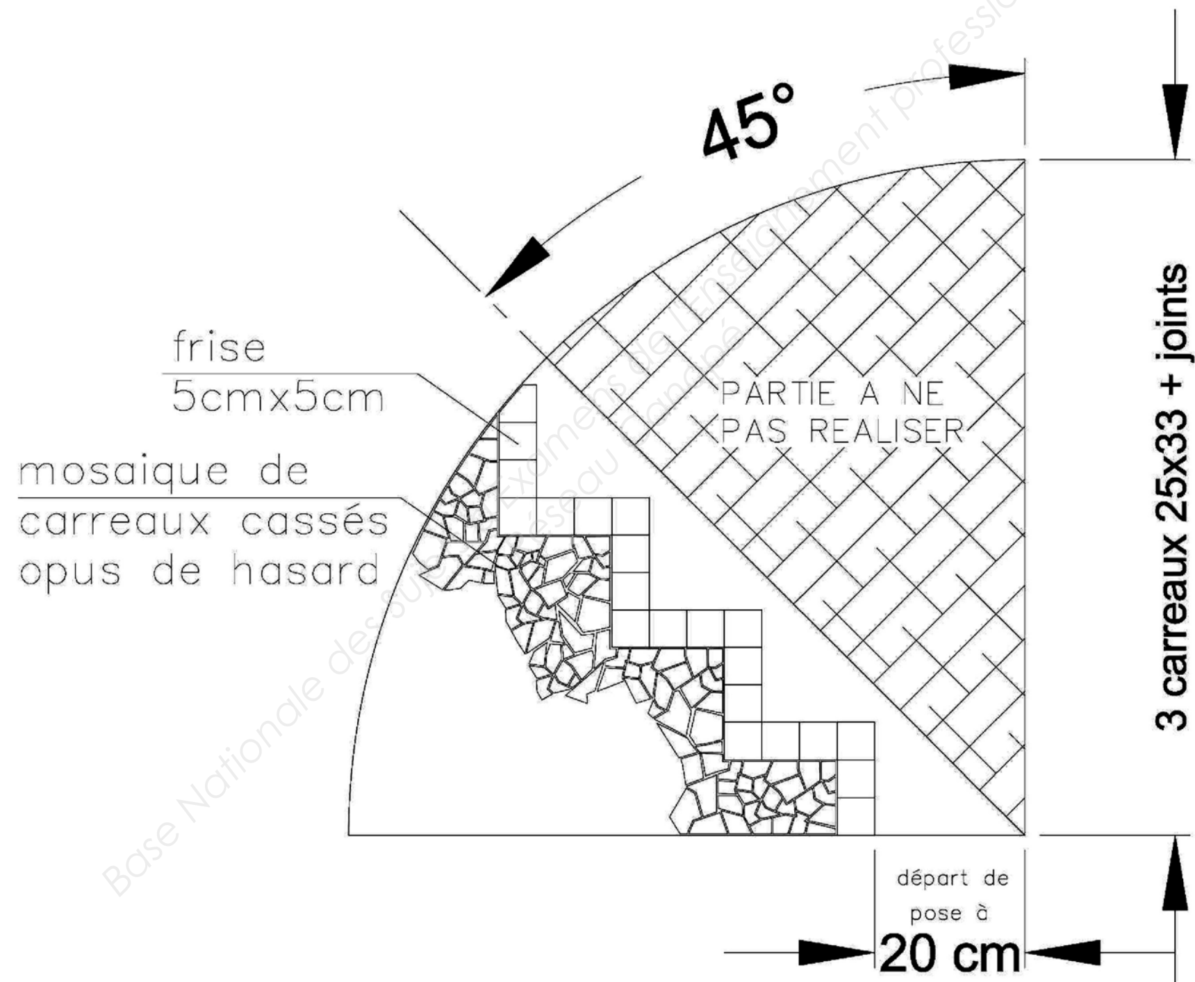
PLAN DE POSE (Échelle indéterminée)
