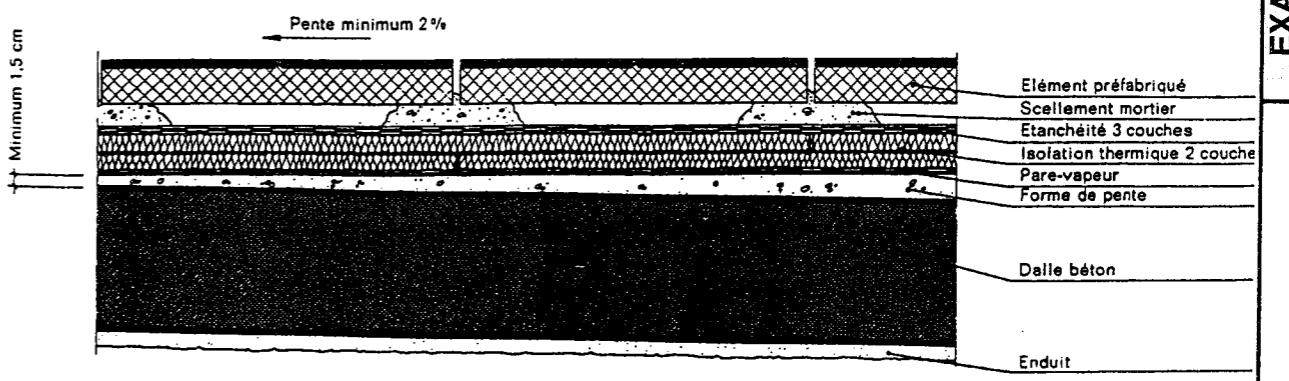
3 Pose d'éléments préfabriqués avec scellement au mortier directement sur isolation.
