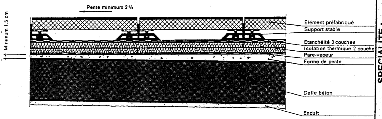
2 Pose d'éléments préfabriqués sur supports réglables en hauteur avec large platine de répartition de charge, directement sur isolation.
